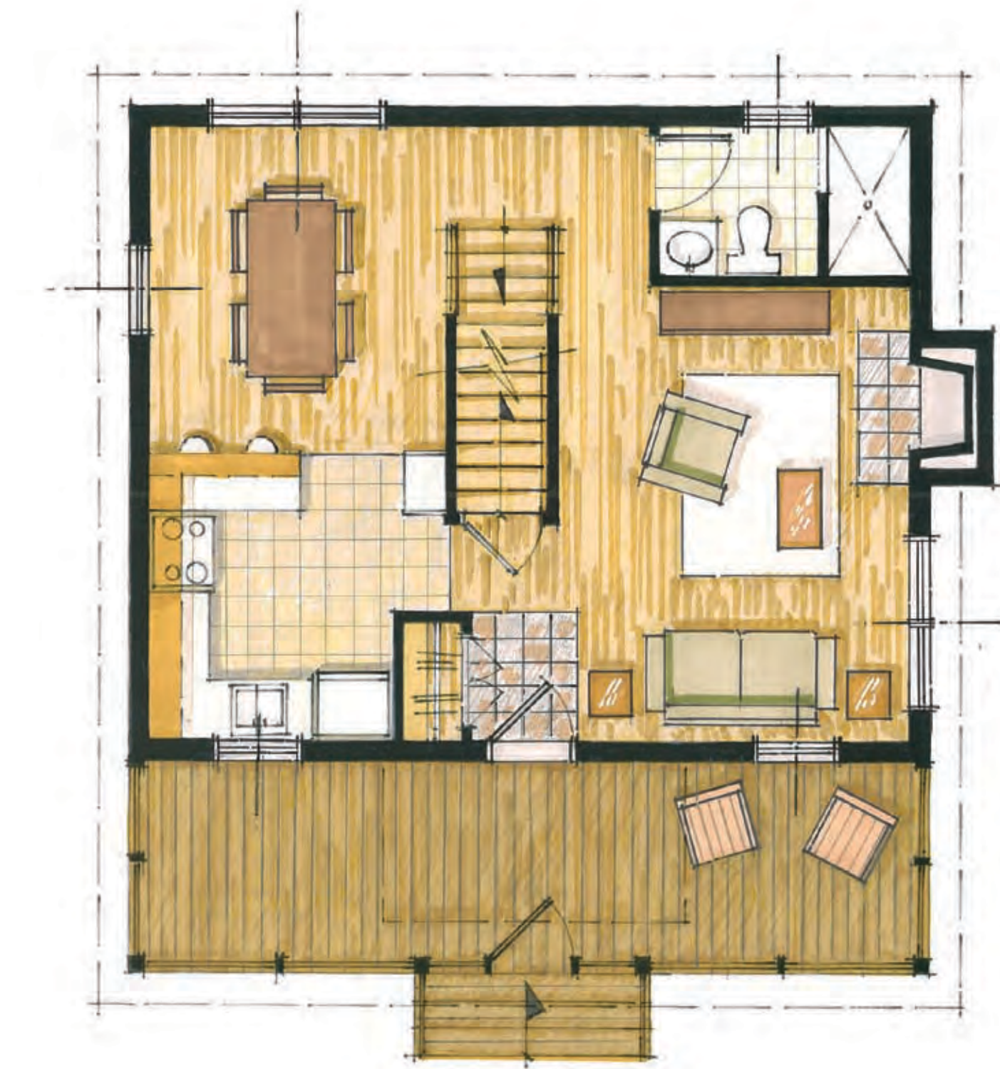
Rez-de-chaussée
