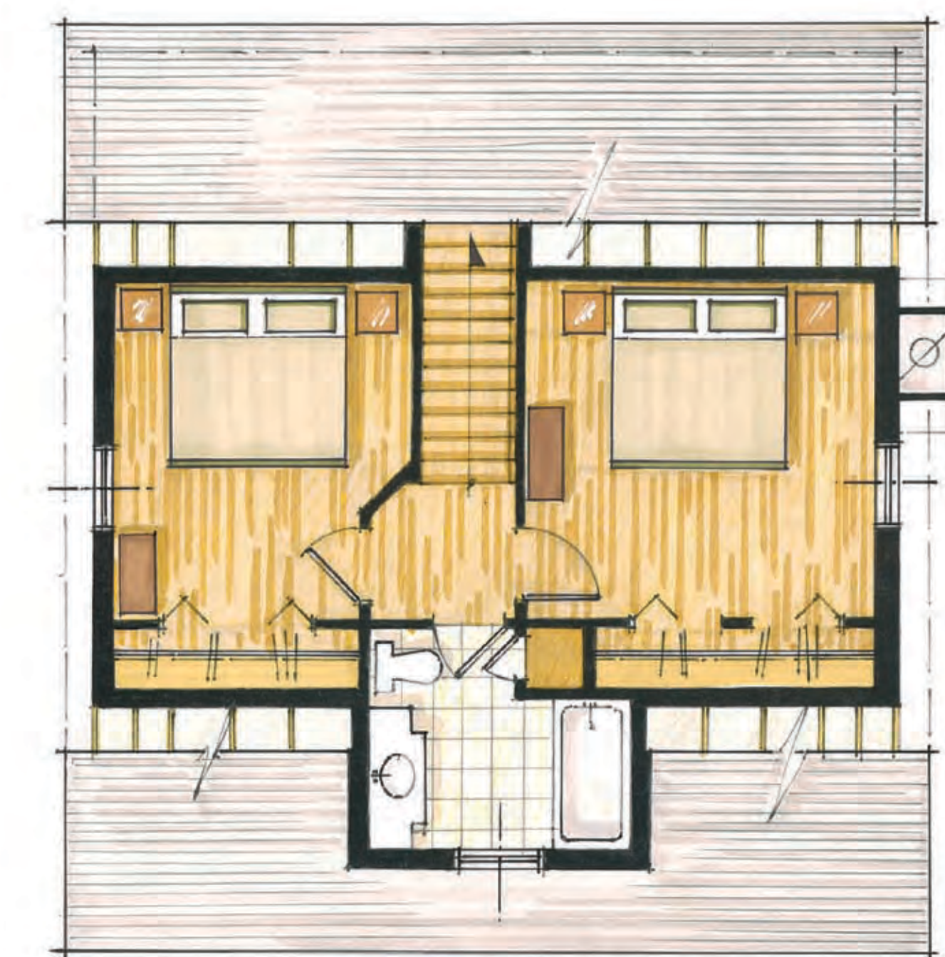
Étage
